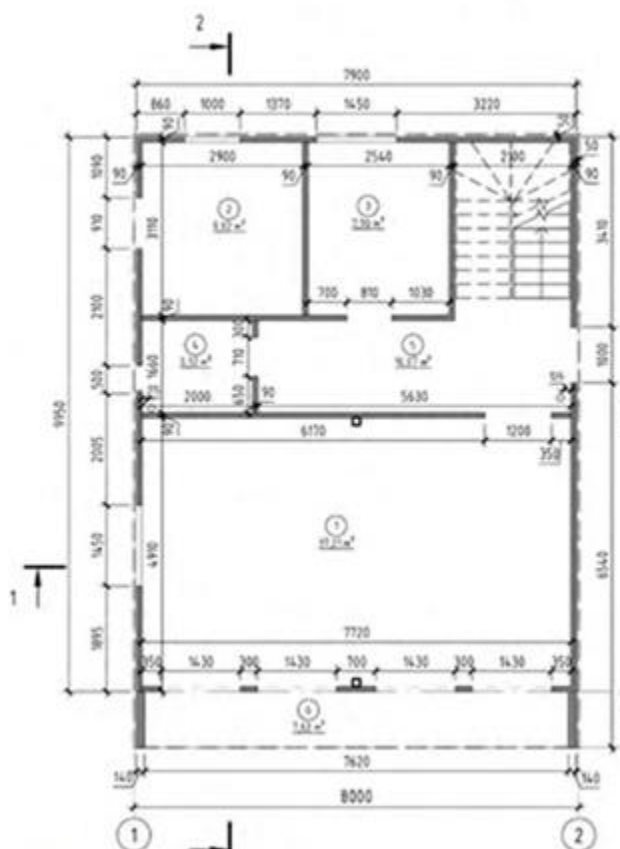
1 этаж М (1: 75)
