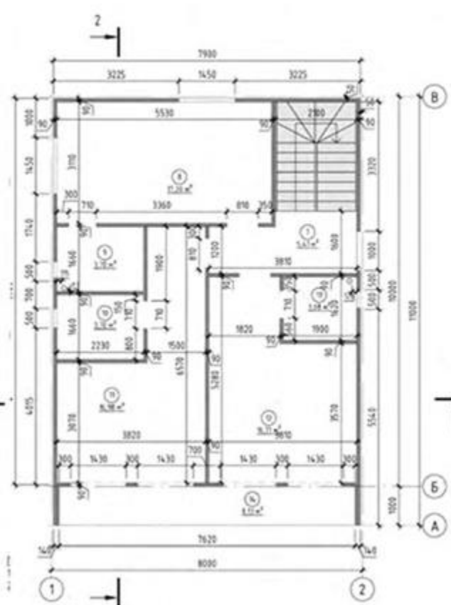
2 этаж М (1: 75)
