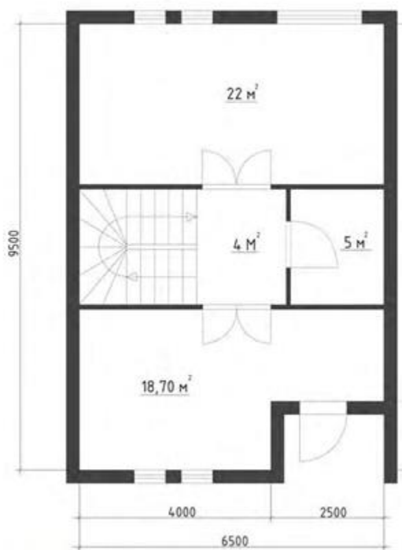
ПЛАН 1 ЭТАЖ
